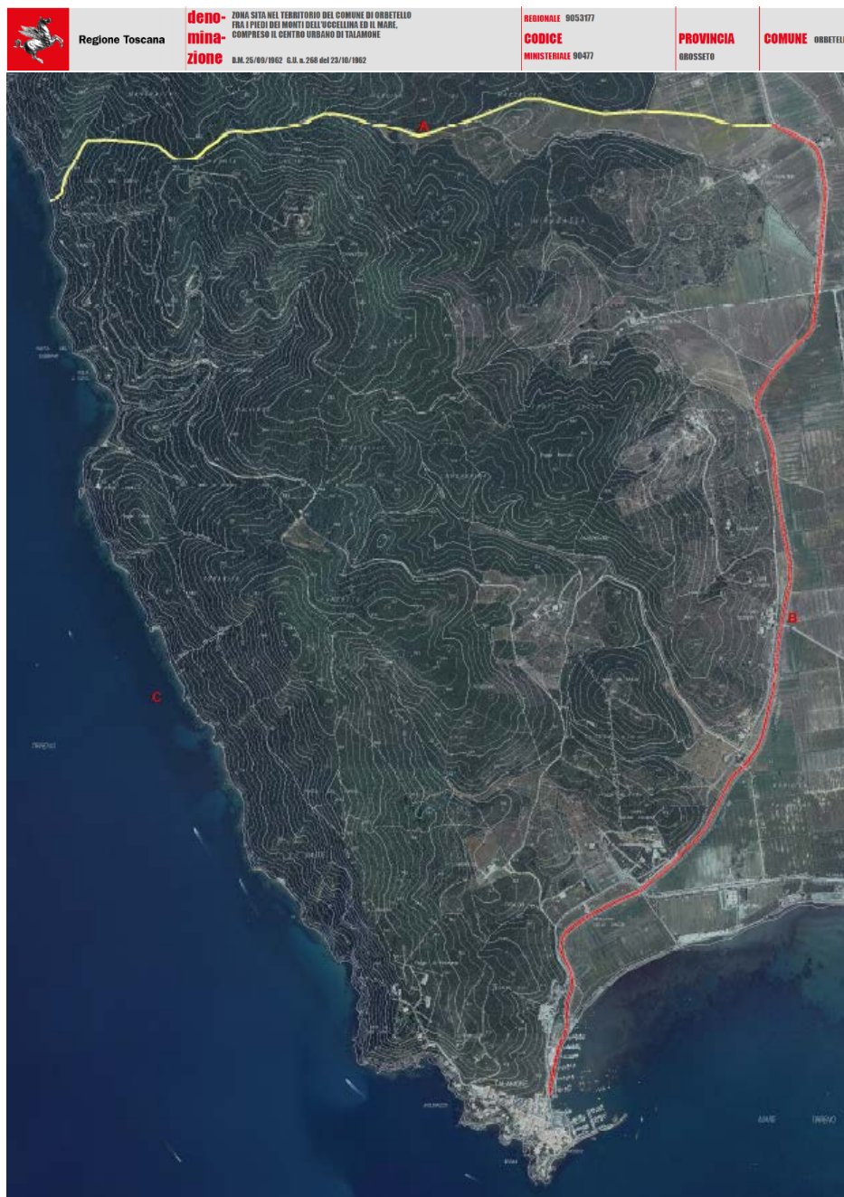
Figura 2 Cartografia - D.M. 25/09/1962 G.U. n. 268 del 23/10/1962
