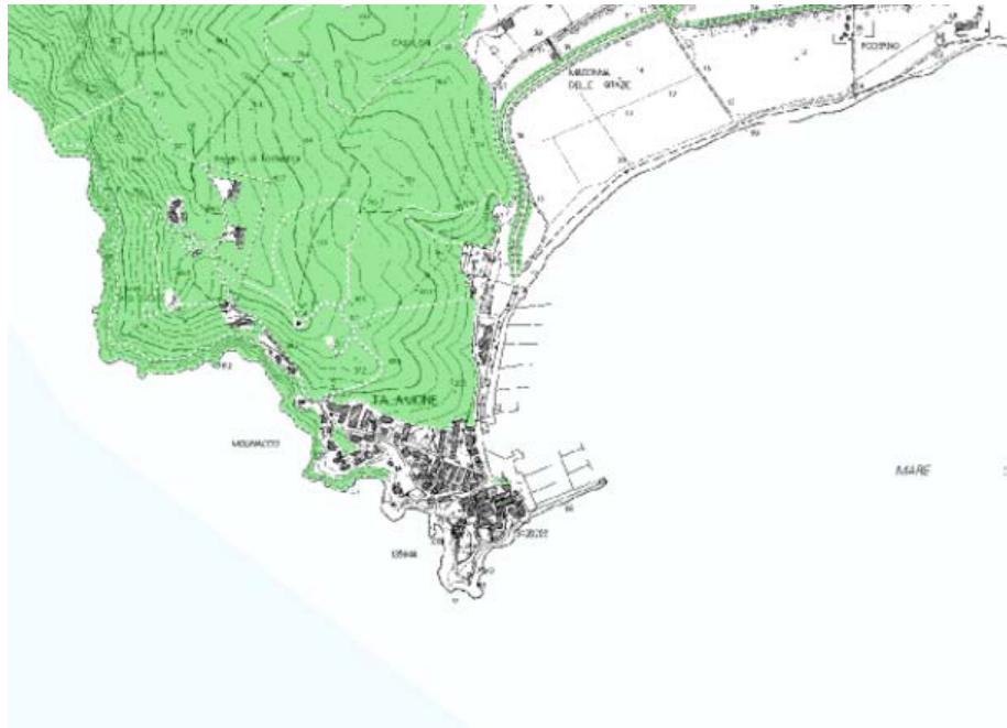
Figura 6 Territori coperti da foreste e da boschi, ancorché percorsi o danneggiati dal fuoco, e quelli sottoposti a vincolo di rimboscimento, come definiti dall'articolo 2, commi 2 e 6, del decreto legislativo 18 maggio 2001, n. 227. (art.142. c.1, lett. g) Codice)
